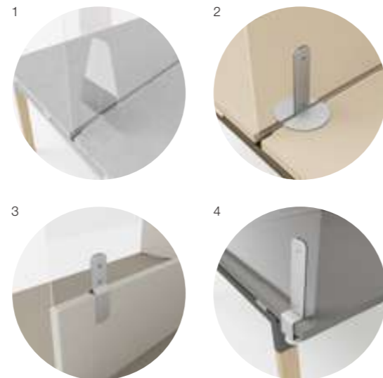
1) Base in metacrilato, 2) Base in metallo, 3) Staffa in metallo, 4) Morsetto in metallo 1) Methacrylate base, 2) Metal base, 3) Metal bracket, 4) Metal clamp 1) Base en méthacrylate, 2) Base métallique, 3) Support métallique, 4) Pince métallique 1) Base de metacrilato, 2) Base metálica, 3) Soporte metálico, 4) Abrazadera metálica
