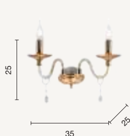
lampadario chandelier AP.CECILIA/2-ORO AP.CECILIA/2A AP.CECILIA/2-TORT power: 2 x E14 voltage: 220-230V
